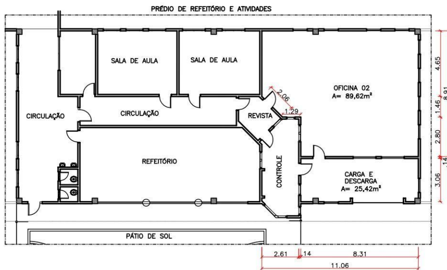
PLANTA BAIXA OFICINA DE TRABALHO 02 Penitenciária Regional de Cachoeiro de Itapemirim - PRCI esc 1:200
