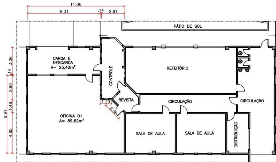
PLANTA BAIXA OFICINA DE TRABALHO 01 Penitenciária Regional de Cachoeiro de Itapemirim - PRCI esc 1:200
