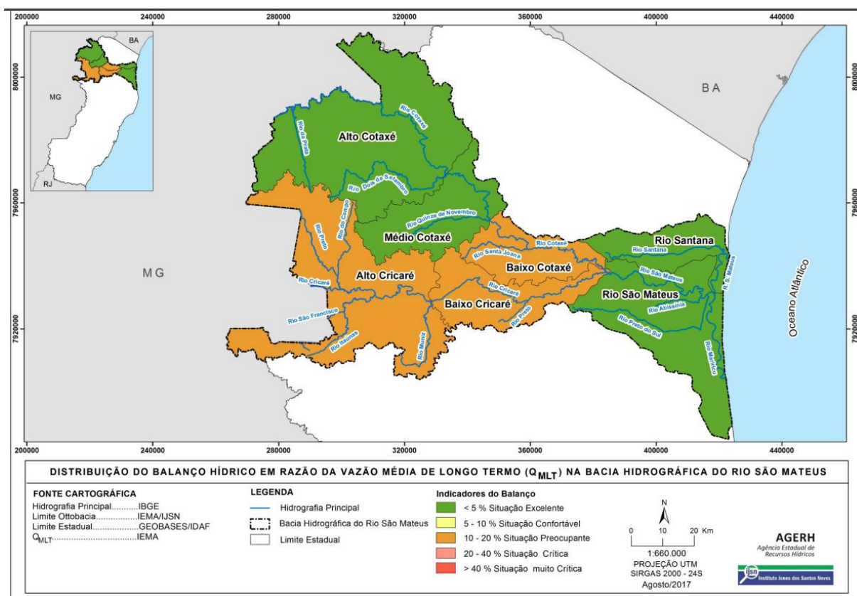
Figura 28: Mapa de distribuição do balanço hídrico na Bacia Hidrográfica do Rio São Mateus – Fonte: Diagnóstico do CBH São Mateus/ AGERH
